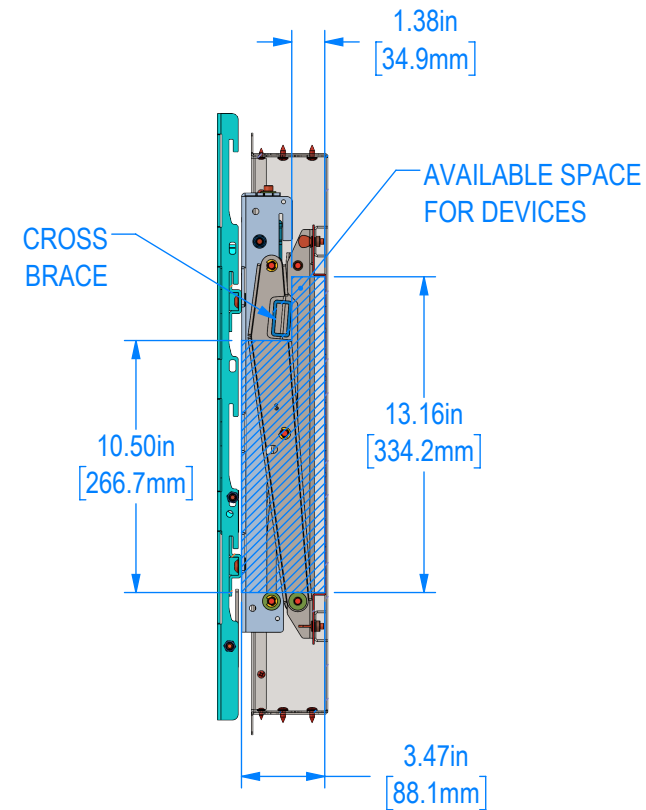
SECTION A-A
